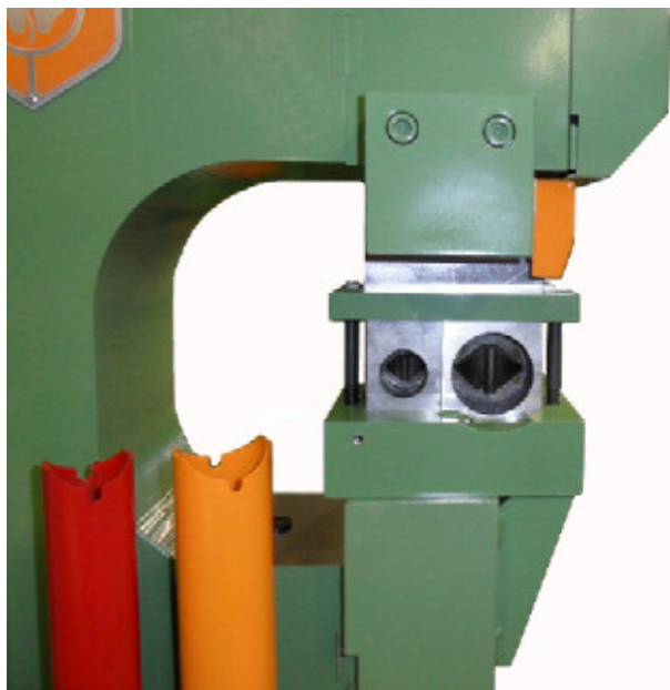
Entallador de tubos cuádruple para la zona de punzondo. Protecciones de dedos eliminadas para la foto.
