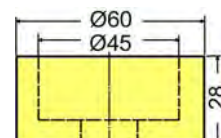
Matrizenreduzierung 60/45 die reducing socket réducteur matrice 10506 063 00 00
