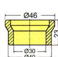
Einsatzbuchse 40/30 punch reducing sleeve réducteur poinçon 10505 315 00 00
