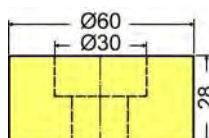
Matrizenreduzierung 60/30 die reducing socket réducteur matrice 10506 062 00 00
