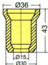
Einsatzbuchse 30/15 punch reducing sleeve réducteur poinçon 10505 313 00 00
