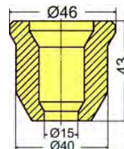
Einsatzbuchse IV/I punch reducing sleeve réducteur poinçon 10505 314 00 00
