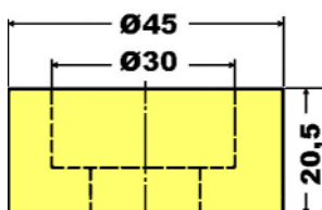
Reduceerinzet 45/30 10506 061 00 00
