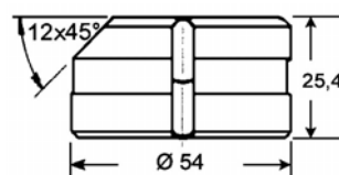
Nr. 271 Matrijs met afgeschuinde zijde
