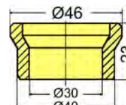
manguito de reducción 40/30 10505 315 00 00
