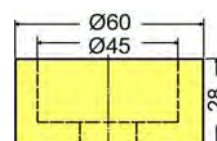
reductor para matriz 60/45 10506 063 00 00
