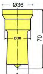
punzón No 52
