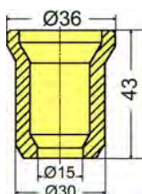
manguito de reducción 30/15 10505 313 00 00
