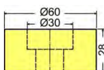
reductor para matriz 60/30 10506 062 00 00
