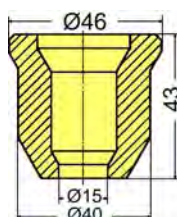
manguito de reducción IV/I 10505 314 00 00
