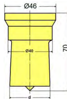
punzón No 53
