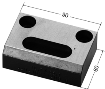
44041 6 3332 03 B Winkelstahlmatrize 317 Langloch quer offset oblong die no. 317 transverse matrice décentrée no. 317, trou oblong sens transversal
