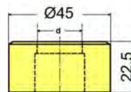
Ø 15,7 – Ø 31,7 mm MBN 50638
