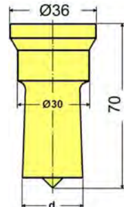
Ø 15,5 – Ø 30,0 mm MBN 50505-2
