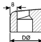
Flanschmatrize offset taper die matrice d'aile
