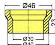
Einsatzbuchse 40/30 punch reducing sleeve réducteur poinçon 10505 315 00 00
