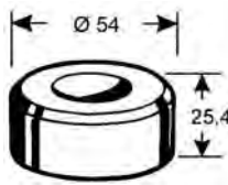
Nr. 271 Matrize die matrice
