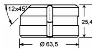
Nr. 291 Matrize mit Schräge die with chamfer matrice à inclinaison
