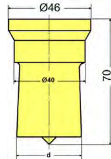
Ø 30,5 – Ø 40,0 mm MBN 50505-3
