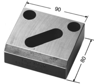
44121 6 2725 02 Winkelstahlmatrize 317, Langloch 45° rechts offset oblong die no. 317, 45° right matrice décentrée 317, trou oblong 45° à droite
