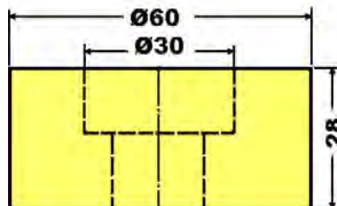
Matrizenreduzierung 60/30 reducing socket réducteur 10506 062 00 00
