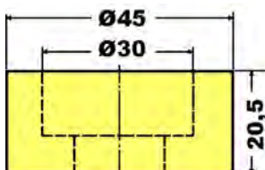
Matrizenreduzierung 45/30 reducing socket réducteur 10506 061 00 00
