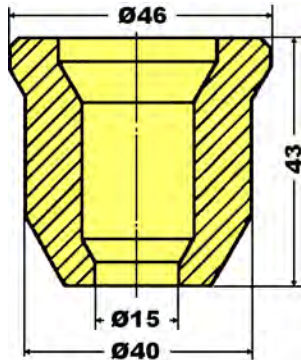
Einsatzbuchse IV/I reducing sleeve réducteur 10505 314 00 00
