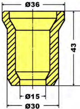
Einsatzbuchse 30/15 reducing sleeve réducteur 10505 313 00 00
