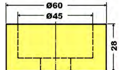
Matrizenreduzierung 60/45 reducing socket réducteur 10506 063 00 00
