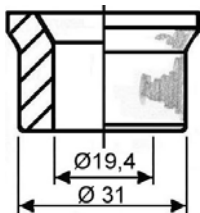
Reduzierhülse 2/5 reducing sleeve réducteur
