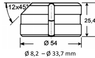
Nr. 271 Matrize mit Schräge die with bevel matrice à inclinaison
