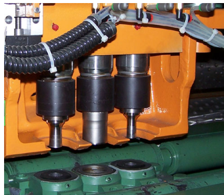
Dreistempel-Werkzeug, schaltbar, für FPDB Triple tool assembly to suit FPDB lines Dispositif de trois poinçons à sélection, pour la ligne FPDB
