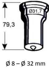
Nr. 272 Stempel punch poinçon
