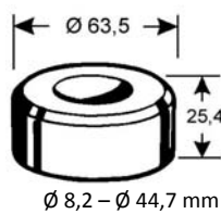
Nr. 291 Matrize die matrice
