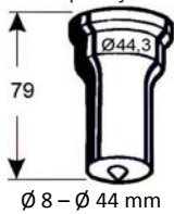
Nr. 292 Stempel punch poinçon
