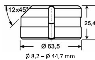
Nr. 291 Matrize mit Schräge die with bevel matrice à inclinaison
