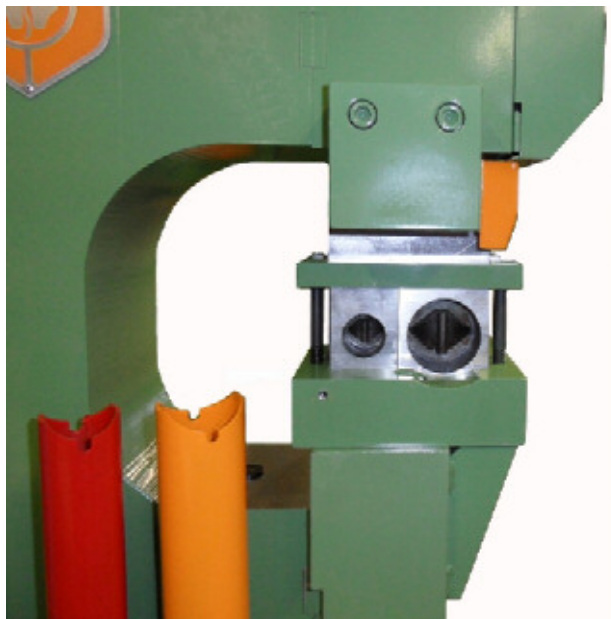
Rohrausklinkvorrichtung, vierfach, unter der Lochstanze. Der Fingerschutz wurde für das Foto entfernt
